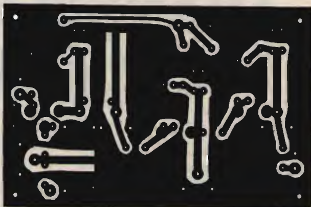
figura 8 Transverter 144/432 MHz, circuito stampato del convertitore trasmittente, lato rame.
