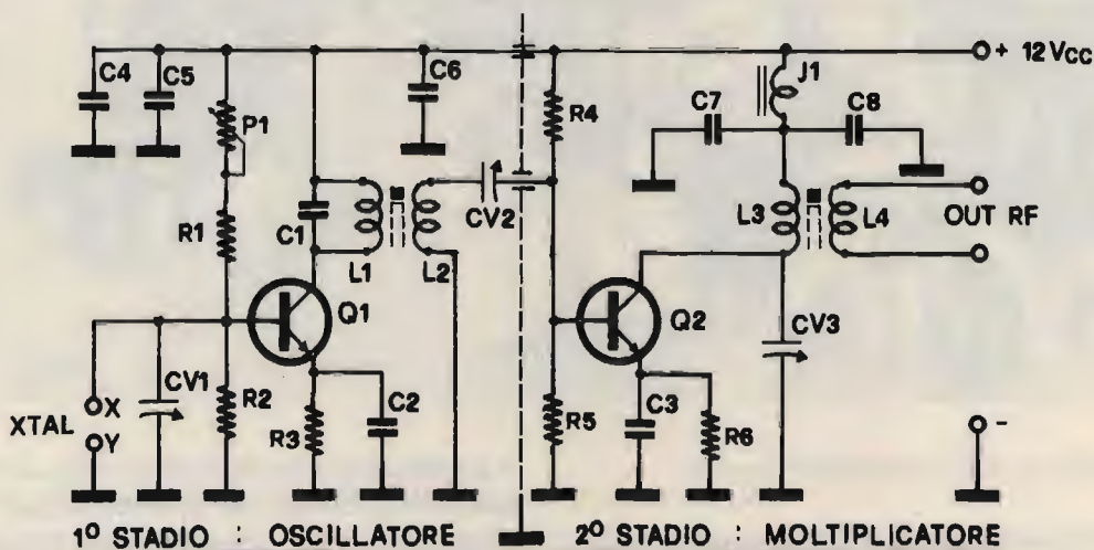
figura 1 Schema elettrico.
