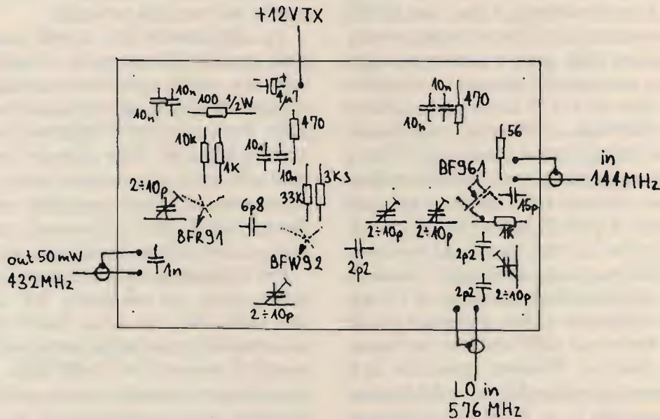
figura 8 bis Transverter 144/432 MHz, disposizione dei componenti del convertitore trasmittente (originale dell'Autore).
