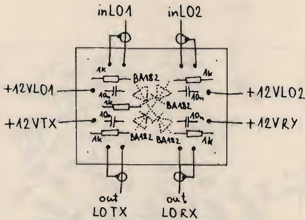
figura 11 bis Transverter 144/432 MHz, disposizione dei componenti della commutazione degli oscillatori locali (originale dell'Autore).
