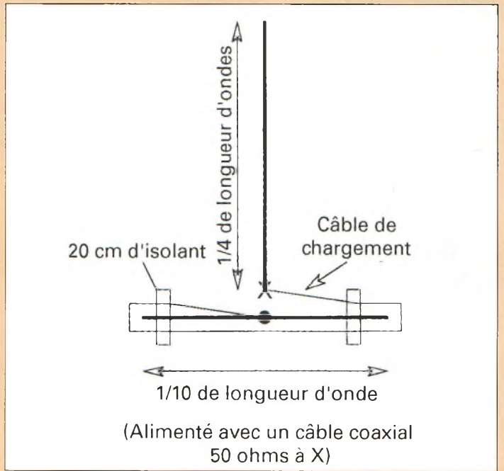
Fig. 8- Système radial en charge linéaire.
