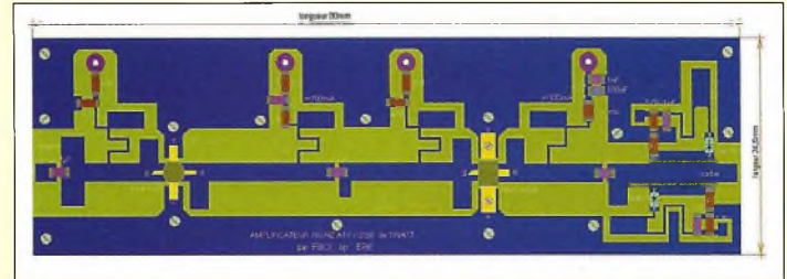
Fig. 10 - L'implantation des composants de l'amplificateur 1 watt.
