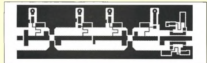
Fig. 12 - Le dessin du circuit imprimé de l'amplificateur 200 milliwatts à l'échelle 1. Vérifiez la longueur qui doit faire 80 millimètres ainsi que les pistes qui font 2 millimètres de large. Notez par ailleurs que l'emplacement du deuxième transistor est plus petit.
