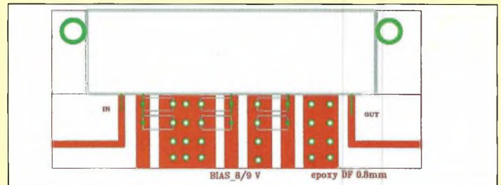
Fig. 5-L'implantation des composants d'un amplificateur hybride. Selon les modèles et les versions, il convient de se reporter au texte pour les brochages.
