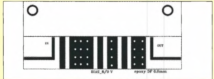
Fig. 4-Le circuit imprimé qui permet de mettre en œuvre les amplificateurs hybrides. Chaque trou correspond à un passage vers la masse.
