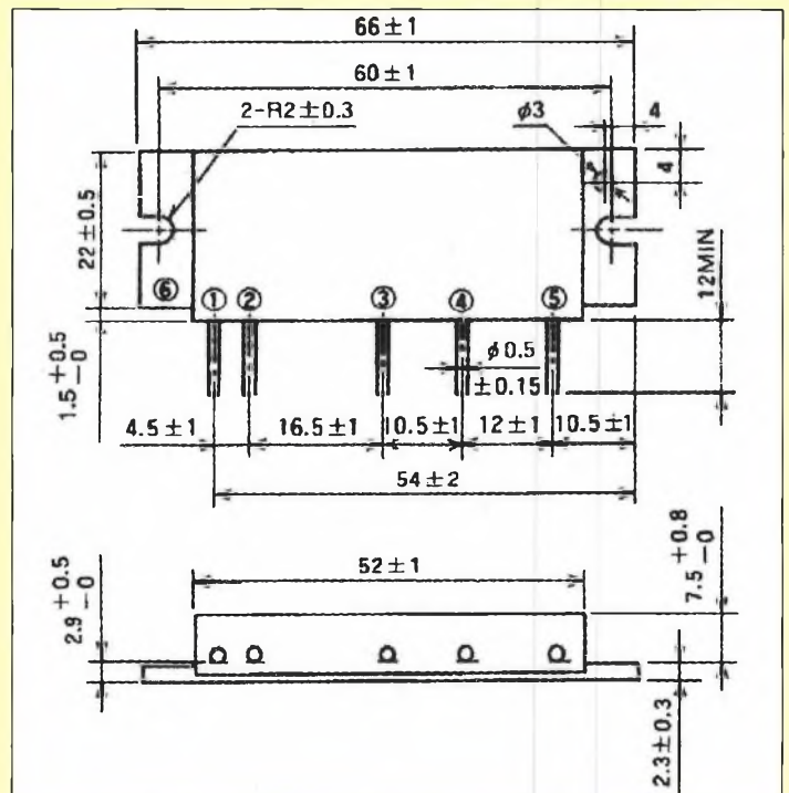
Fig. 6-Les dimensions des hybriques à 5 broches.
