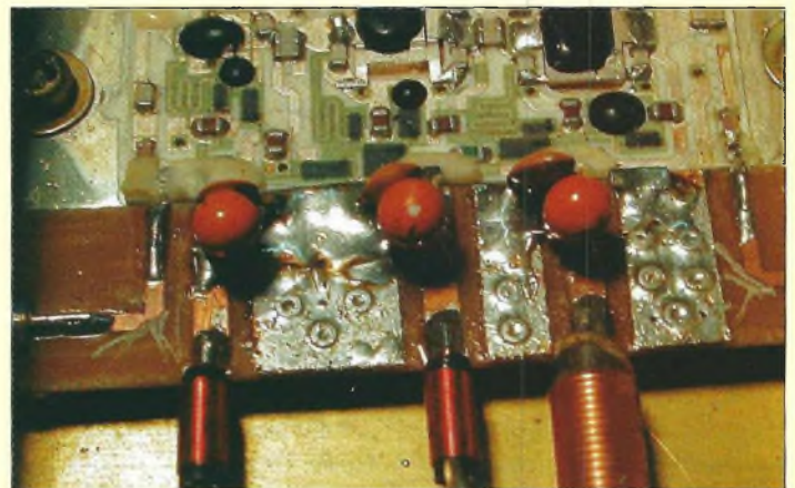
Fig. 16-Un amplificateur hybride sur 1200 MHz. Il convient de placer un feuillet sous le sabot de l'hybride pour faire venir la masse sur le dessus du circuit imprimé.
