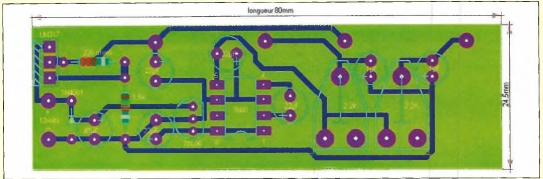
Fig. 14-L'implantation des composants de l'alimentation.
