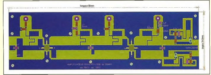
Fig. 9 - L'implantation des composants de l'amplificateur 200 milliwatts.
