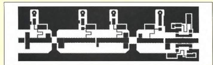
Fig. 11 - Le dessin du circuit imprimé de l'amplificateur 1 watt à l'échelle 1. Vérifiez la longueur qui doit faire 80 millimètres ainsi que les pistes qui font 2 millimètres de large.
