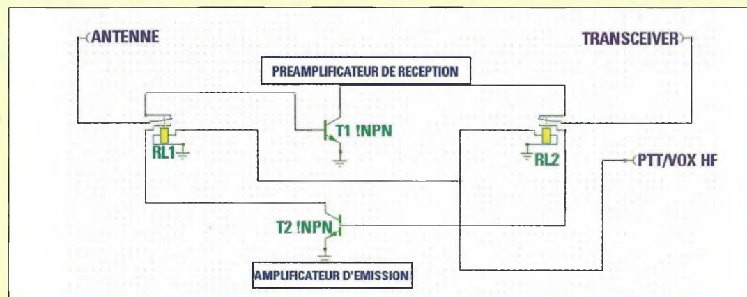
Fig. 1-Le synoptique représentant le fonctionnement global d'un amplificateur que l'on raccorde directement sur la prise antenne d'un transceiver.
