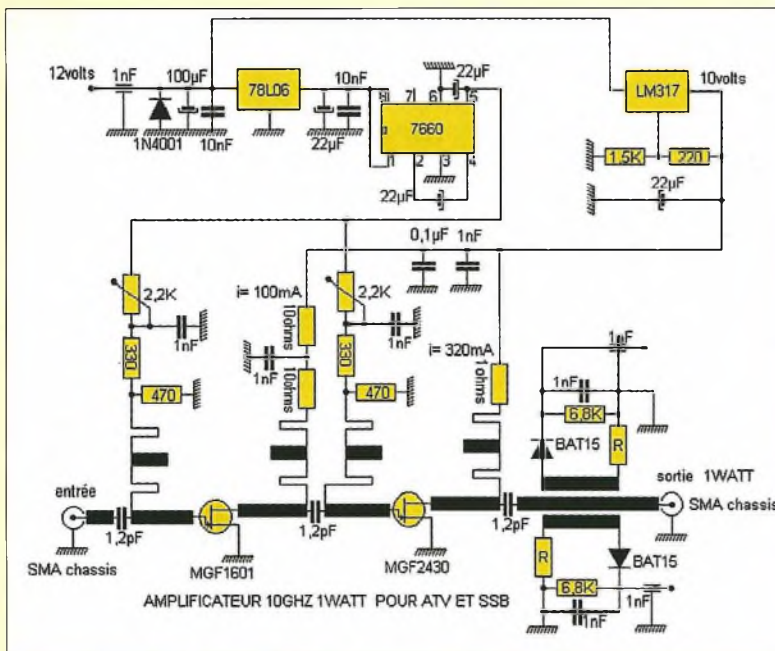
Fig. 8 - Le schéma électrique de l'amplificateur linéaire sur 10 giga et de son alimentation.
