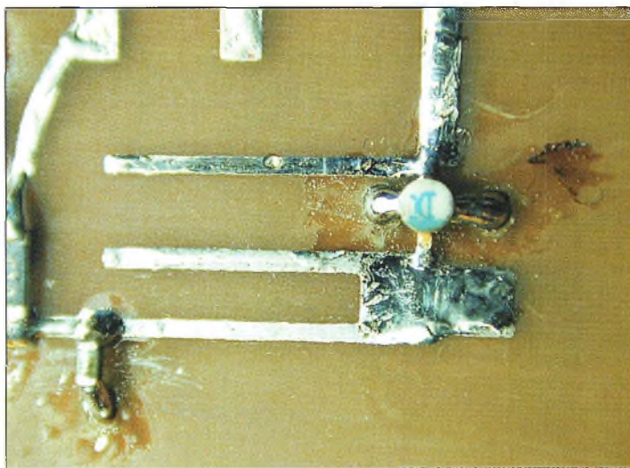
Les soudures paraissent délicates vu les faibles espacements des lignes couplées.
