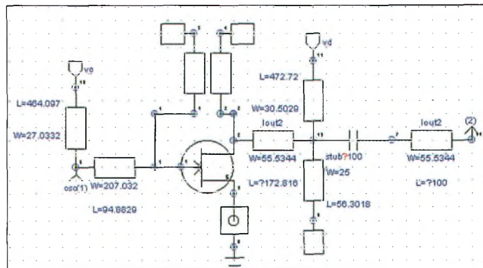
Figure 1—Le schéma de principe de l'oscillateur libre sur 10 GHz.
