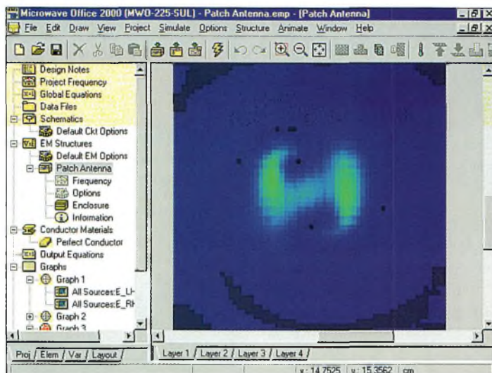
Fig. 1 - Les courants en bleu se propagent dans le patch du centre vers les bords en forme de spirale. Cette antenne est attaquée sur l'un de ses quatre coins.
