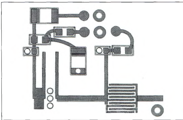
Figure 4-L'implantation des composants de l'oscillateur à l'échelle 2.
