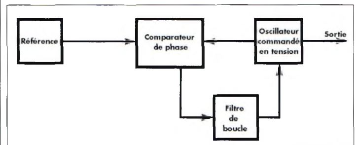
Fig. 4- Une boucle à verrouillage de phase (PLL) classique.
