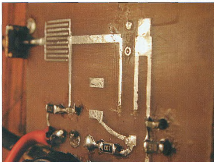
Notez les rivets en cuivre qui viennent à fleur de la surface supérieure du circuit imprimé.
