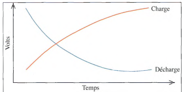
Fig. 2- Courbe de charge et de décharge d'un condensateur dans le temps.
