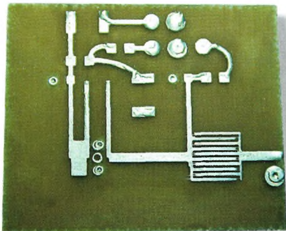
Le circuit imprimé une fois l'étamage réalisé.
