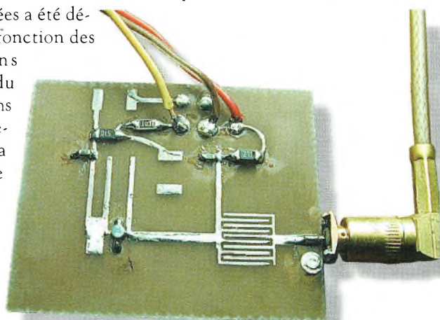
Dans la version de base, une tension négative était nécessaire. Le fil jaune l'amenait.
