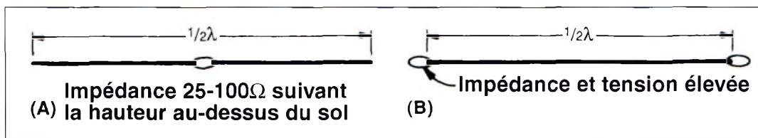
Fig. 4- En (A), un dipôle demi-onde alimenté au centre. Au point d'alimentation, l'impédance est voisine de 50 ohms, ce qui autorise l'emploi d'un câble coaxial. En (B), une antenne Zepp. Il s'agit toujours d'une demi-onde, mais cette fois alimentée à une extrémité. L'impédance est passée à quelque 4 000 ohms, d'où la nécessité d'adopter une ligne d'alimentation de type bifilaire, symétrique. La tension est très élevée aux extrémités de l'antenne.
