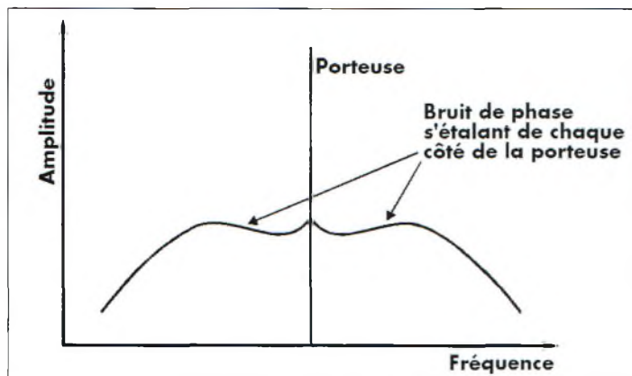
Fig. 2- Caractéristique du bruit de phase d'un synthétiseur typique à une seule boucle.
