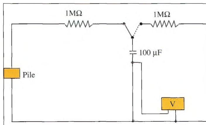
Fig. 1- Un circuit simple pour comprendre le fonctionnement d'un condensateur.
