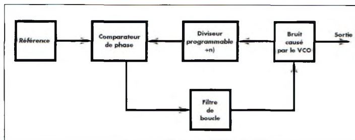
Fig. 5- Schéma d'un synthétiseur de fréquences utilisant un diviseur programmable dans la boucle.
