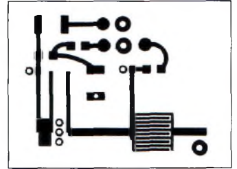
Figure 3- Le dessin du circuit imprimé à l'échelle 1.
