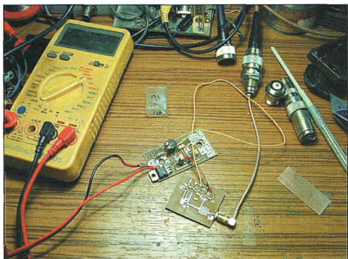
Les premières manipulations avec le circuit proposé ce mois-ci, équipé d'un transistor ATF132B4, 10 mW à la clef.
