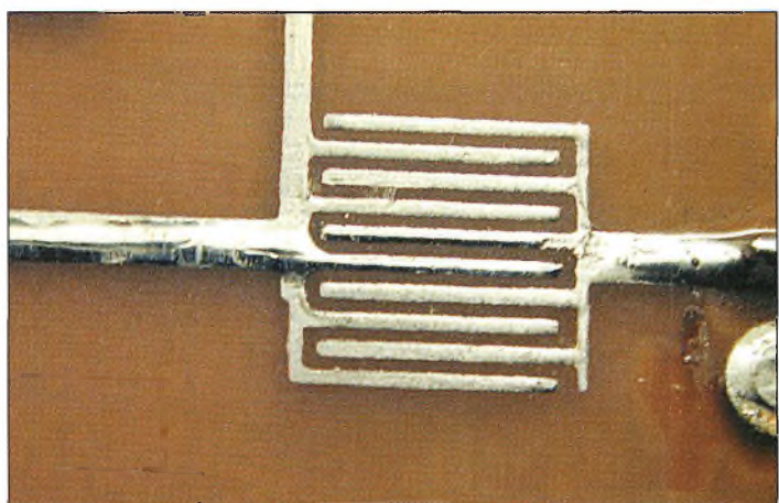
Le peigne de sortie nécessite beaucoup d'attention lors de la gravure au perchlore de fer.
