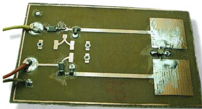
Photo 1- Un oscillateur 10 GHz basé sur une antenne patch.
