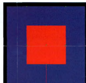
Fig. 2- Le dessin d'un patch sur 1 255 MHz avec l'adaptation quart d'onde.
