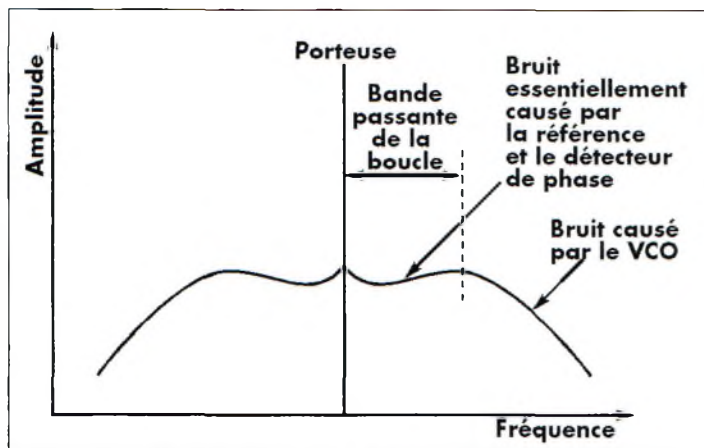
Fig. 6- Formation du bruit dans un synthétiseur.
