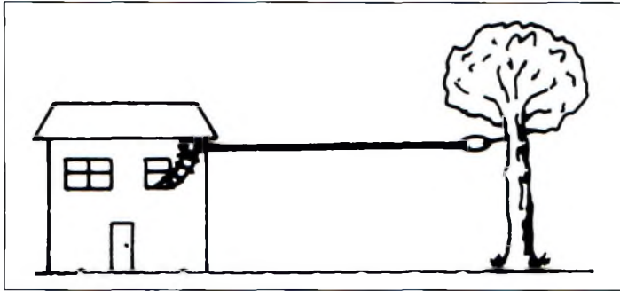
Fig. 3- Une installation typique de l'antenne Zepp.
