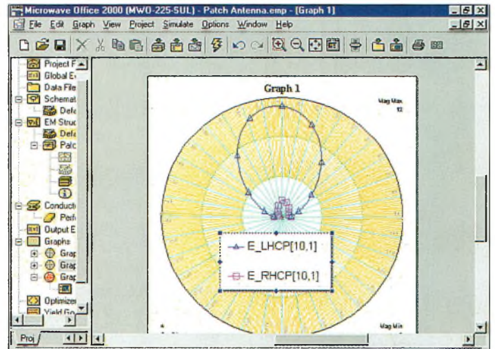
Fig. 4- La directivité de l'antenne simulée (voir la fig. 1).
