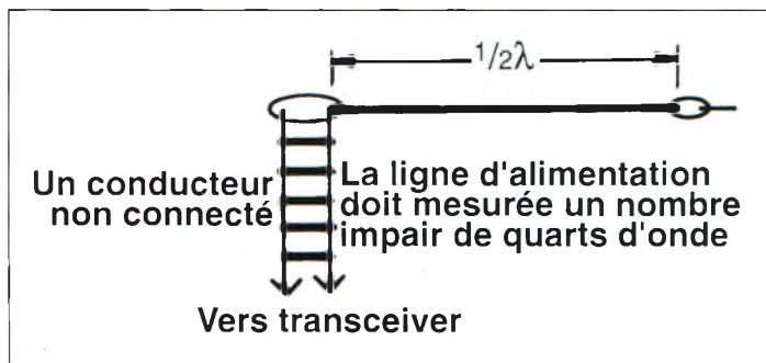
Fig. 2 - L'antenne Zepp est un fil d'une demi-onde alimentée par une ligne bifilaire d'impédance élevée (450 ohms par exemple). L'un des conducteurs de cette ligne n'est pas relié, ni à l'antenne, ni à l'émetteur.
