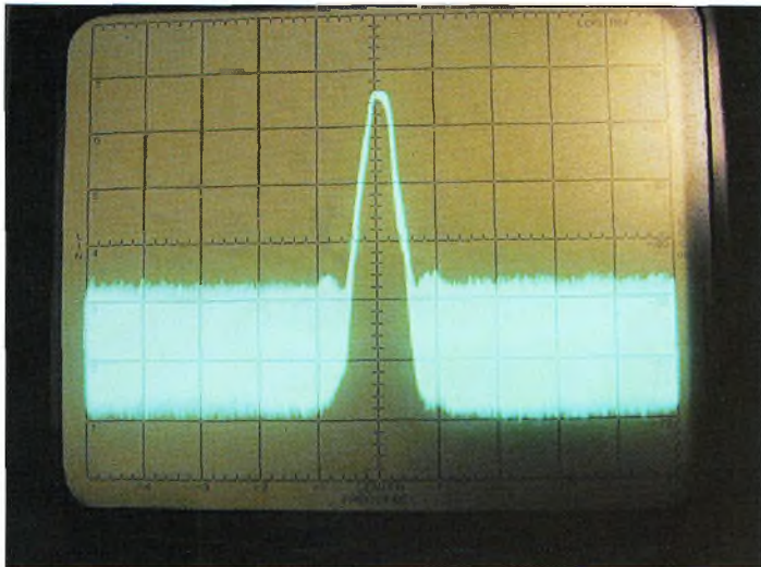
La raie spectrale obtenue avec le transistor ATF13284, la fréquence était de 9 900 MHz. La ligne de référence supérieure est calibrée sur "+20 dBm".
