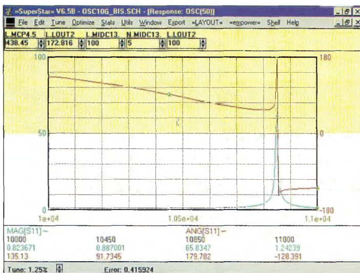
Figure 2 - Les courbes de déphasage et d'adaptation en entrée du transistor FET.
