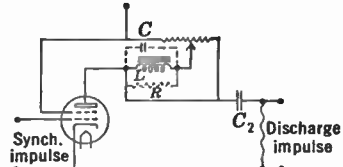
FIG. 15.21.—Dynatron Oscillator.
