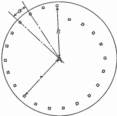
FIG. 8.1.—Nipkow Disk.
