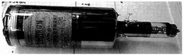
Emitron. Dave Johnson photo.
