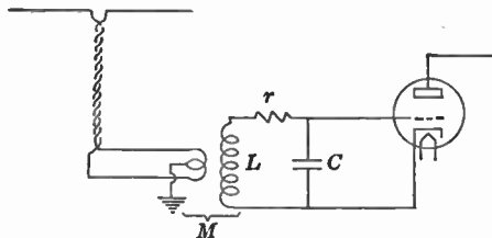
FIG. 17.7.—Simple Input Circuit.
