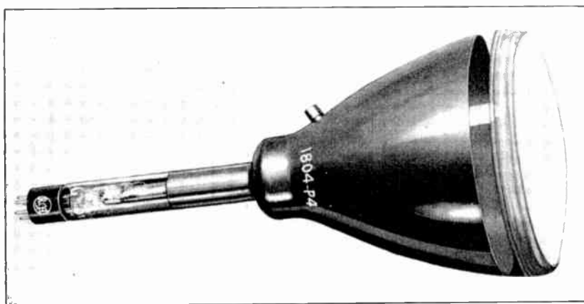
FIG. 12.19.—Nine-Inch Kinescope (RCA 1804-P4).
