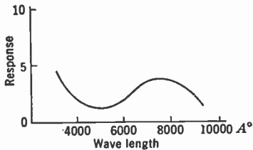
FIG. 1.13.—Spectral Response of Cs-CsO-Ag (Zworykin and Wilson).
