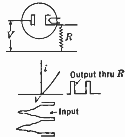
FIG. 15.29—Diode Separator.
