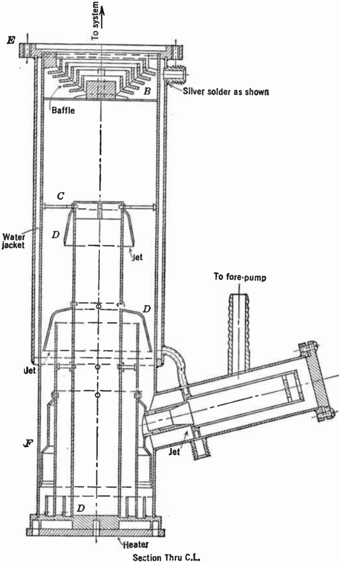
FIG. 5.8.—Oil Diffusion Pump.
