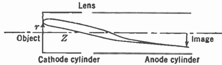
FIG. 4.17.—Cathode Lens.
