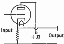
FIG. 15.30.—Cathode-Follower Separator.
