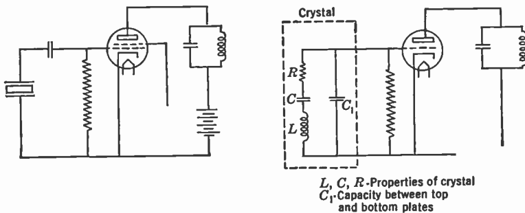
Fig. 16.5.—Crystal Oscillator.
