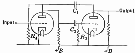
FIG. 15.35.—Multivibrator.
