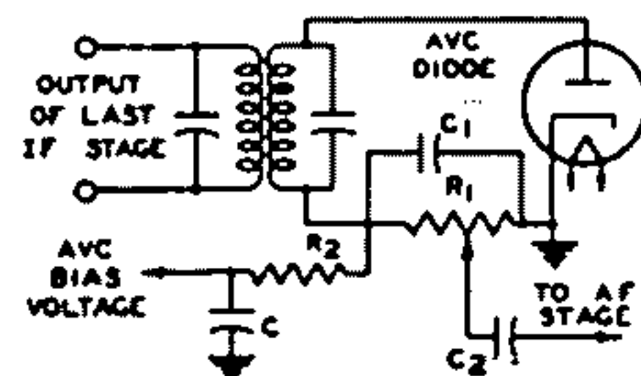
Fig. 61—Automatic-volume-control (avc) circuit.
