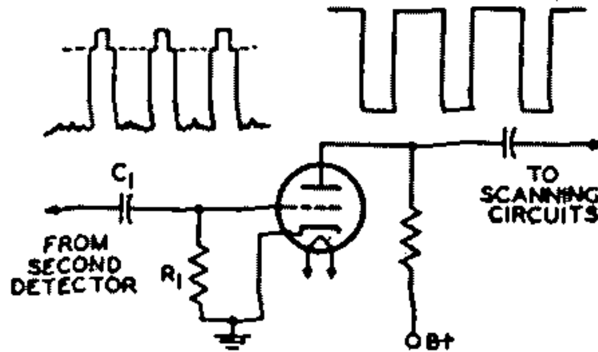
Fig. 80—Sync-separator circuit.
