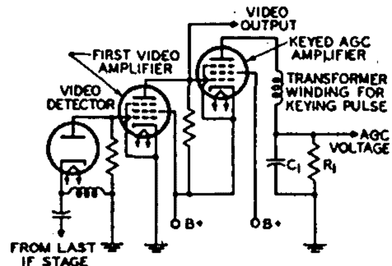
Fig. 64—"Keyed" agc circuit.
