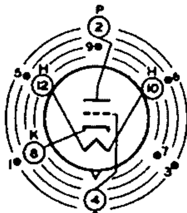
INDEX=LARGE LUG ●=SHORT PIN—IC
