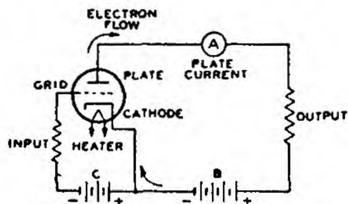
Fig. 6—Basic triode circuit.
