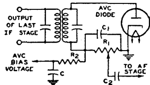
Fig. 67—Automatic-volume-control (avc) circuit.
