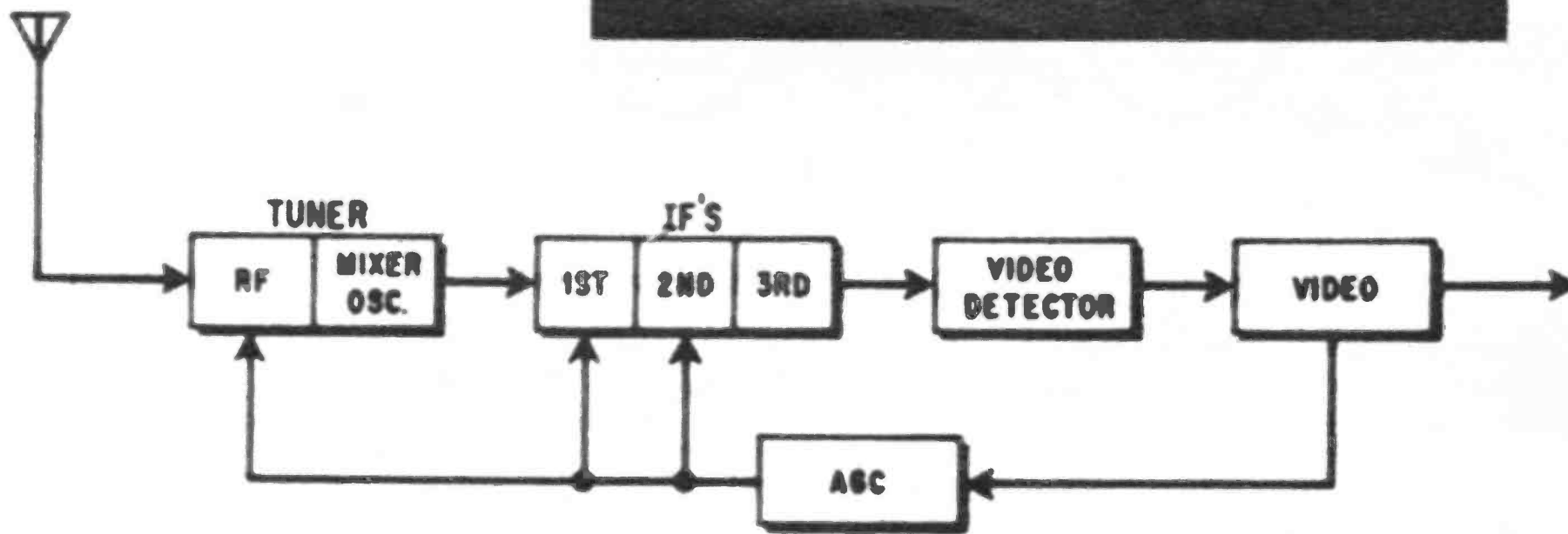
AGC FEEDBACK
