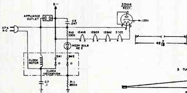
Filament Wiring
