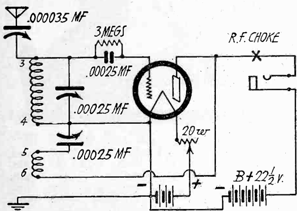
Fig. 1. Schematic Wiring Diagram
