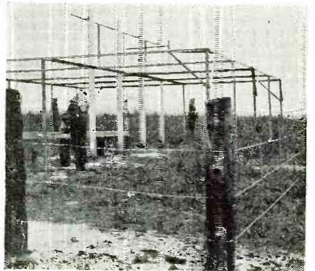
Fig. 9. Fan marker antenna installation.
