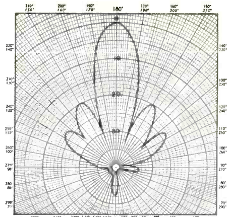
Fig. 3. H-plane pattern for 6' antenna.
