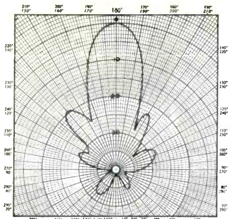
Fig. 2. E-plane pattern for 6' antenna.
