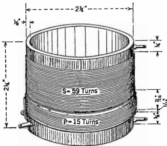
No 24 D.S.C. Wire
