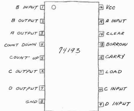
Fig. 4. 74193 pin diagram.
