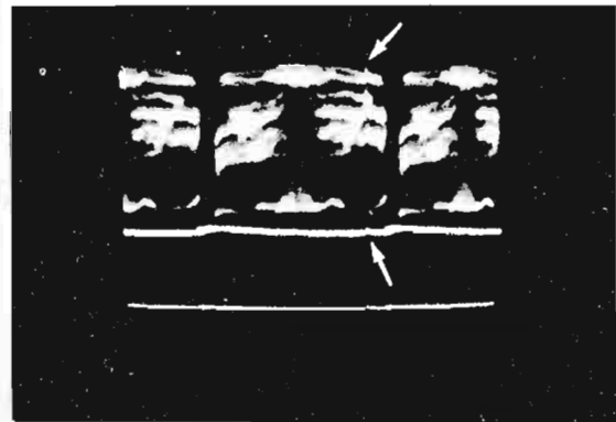
Fig. 121. Glitch—vertical.
