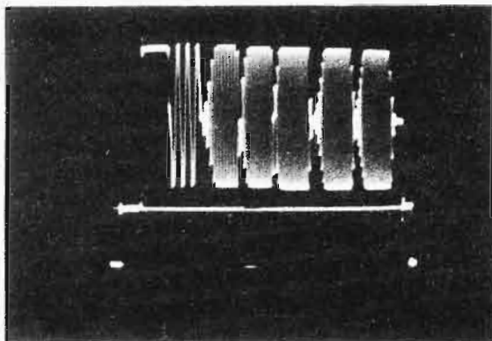
Fig. 22. Multiburst signal—horizontal.
