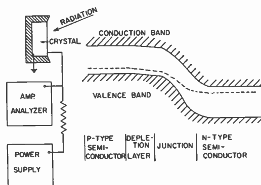
Fig. 3—Semiconductor detector.
