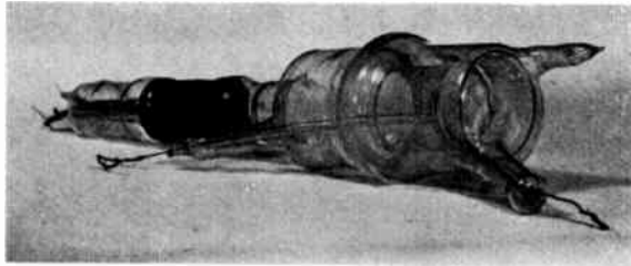
Fig. 3—Prototype of storage-type camera tube (Zworykin, 1923).
