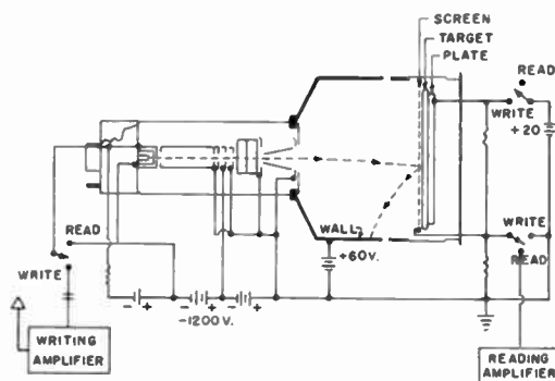
Fig. 10—Radechon tube (RCA).
