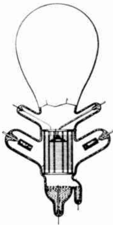
Fig. 4—Langmuir's thyatron.
