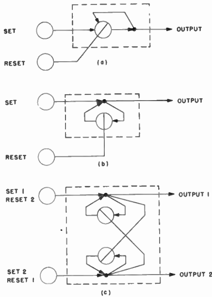
Fig. 11—Flip-flops.
