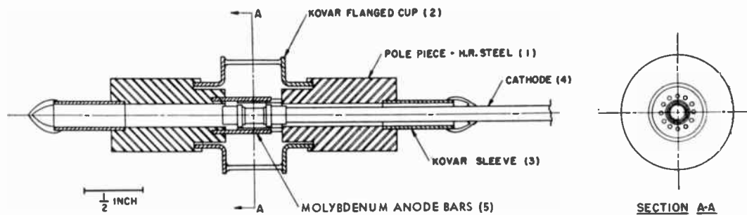
Fig. 2—Mitron.
