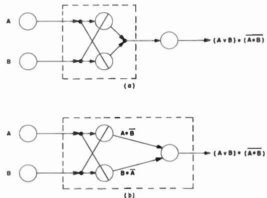
Fig. 9—Exclusive OR.
