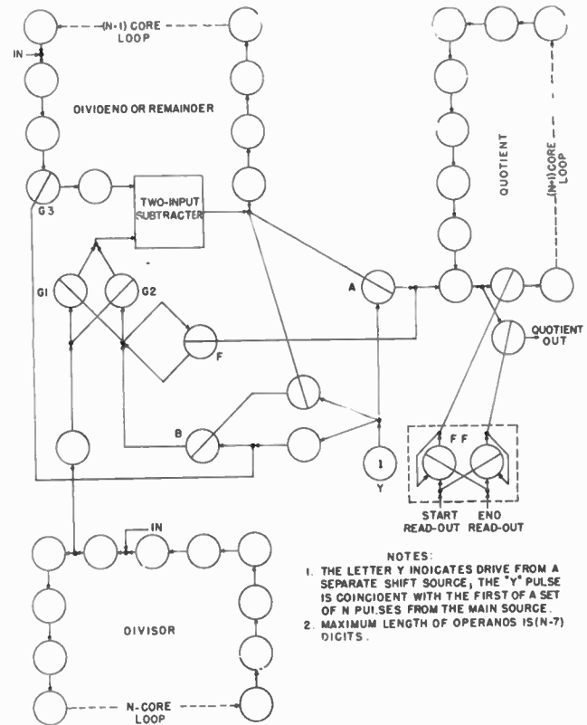
Fig. 19—Divider.
