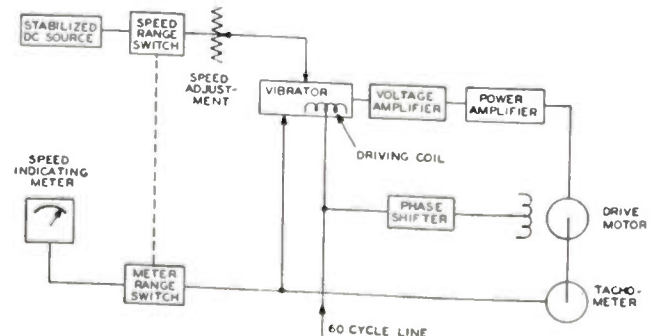
Fig. 6—Block diagram.
