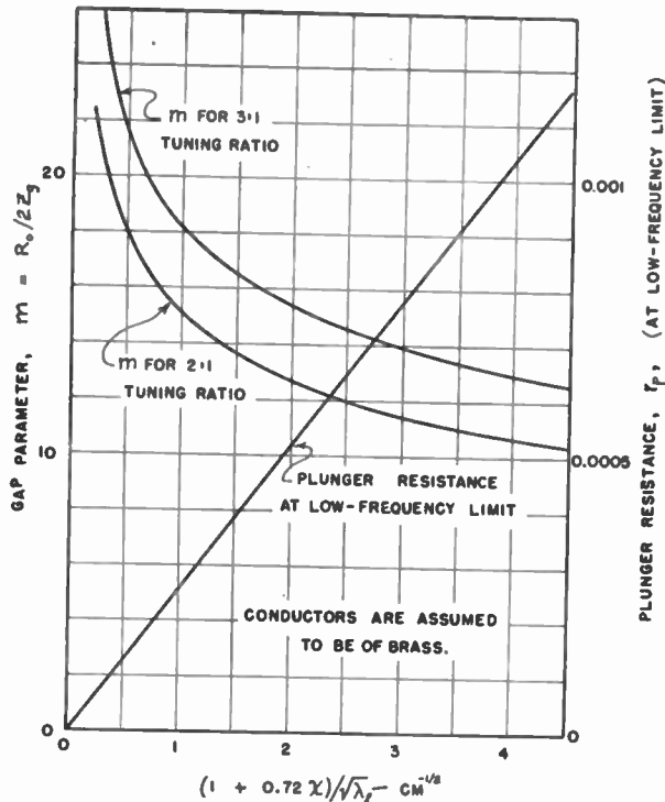
Fig. 8—"Optimum" design data.
