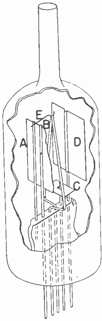
Fig. 1—The ionization gauge.
