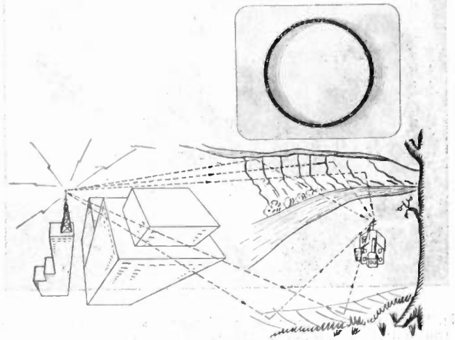
Fig. 14—Type B—smear ghost.
