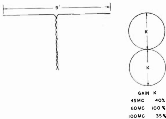
Fig. 1—Horizontal dipole.
