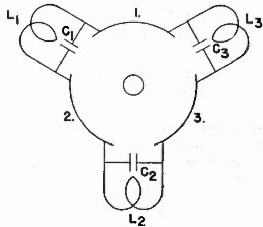
Fig. 15—A 3-phase magnetron.
