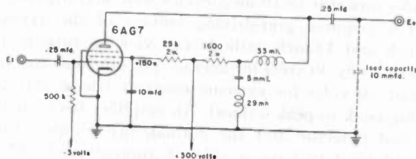
Fig. 18—10-megacycle amplifier.
