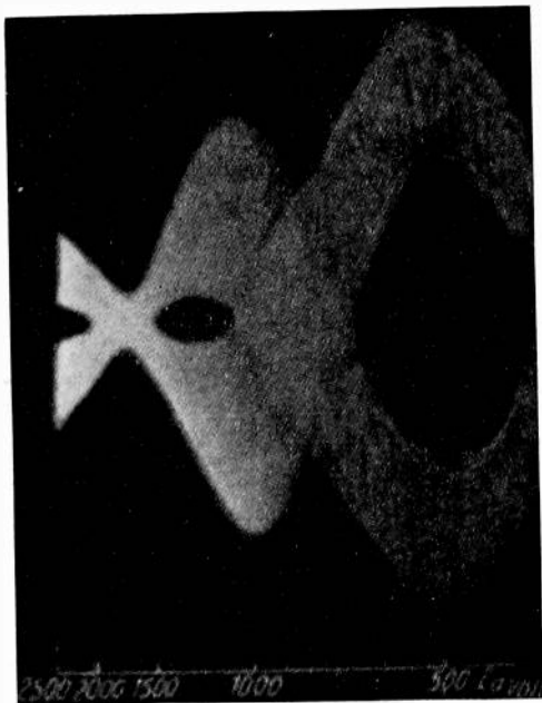
Fig. 5—Overmodulation spectrum.
