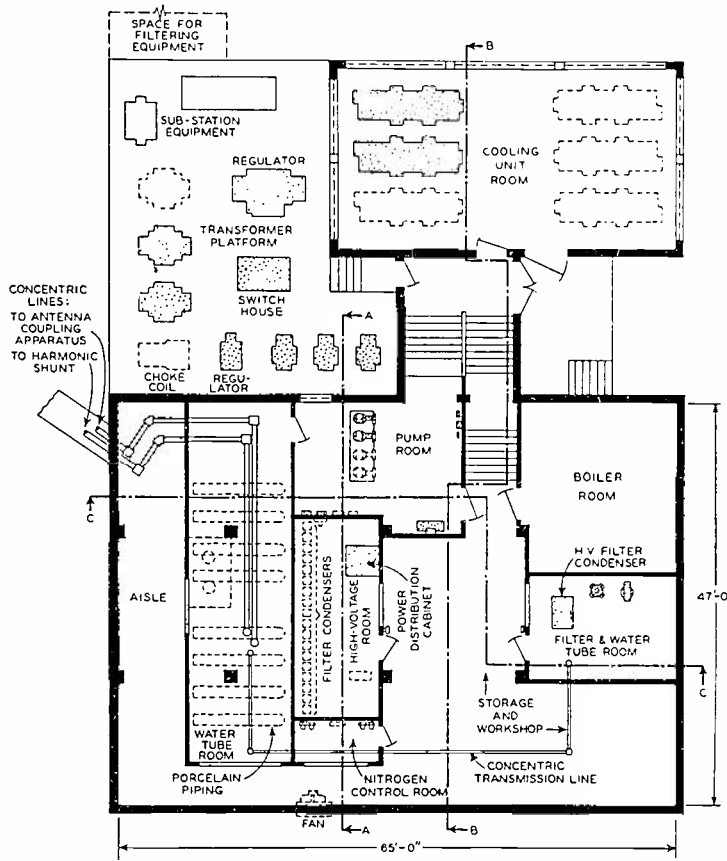
Fig. 2--Basement-floor plan.
