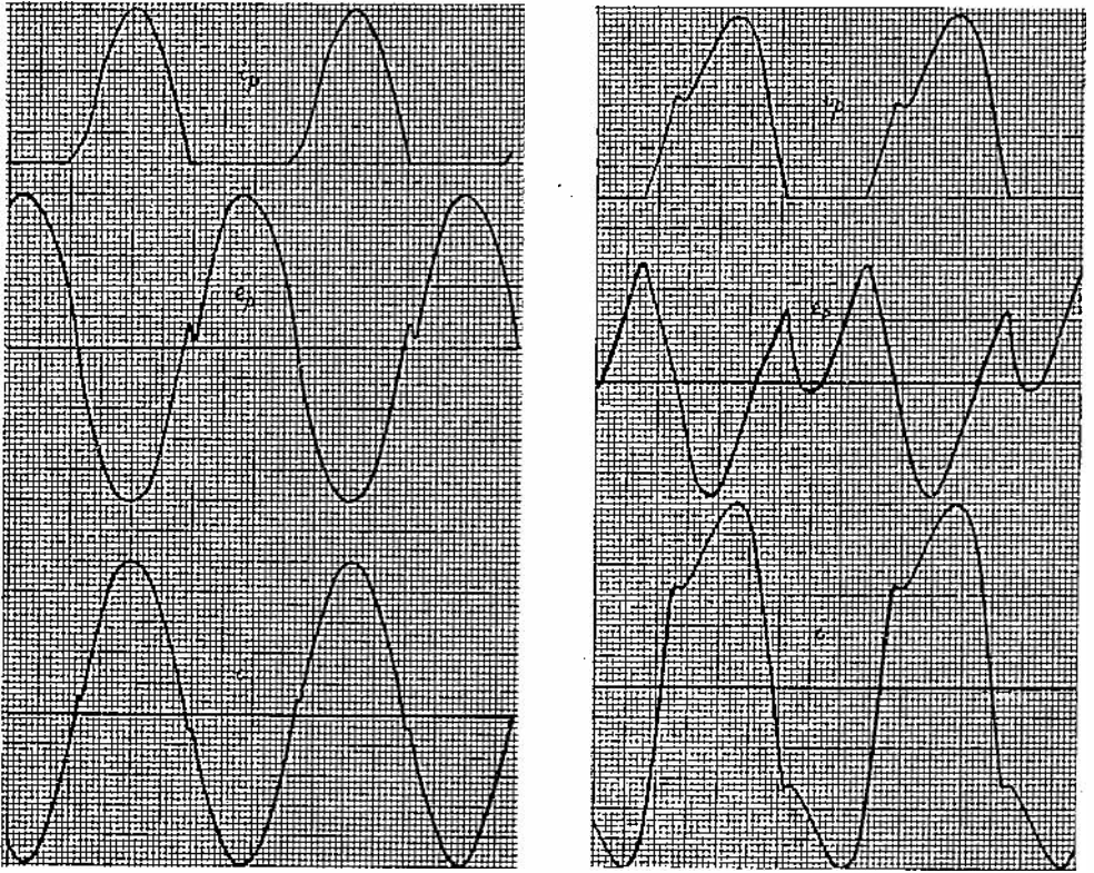
Fig. 6— r = \rho = 4\omega L_1 ; 2L_2 = L_1 ; m = 4 ; n = 16 .
