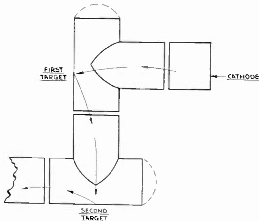
Fig. 15—T type multiplier.
