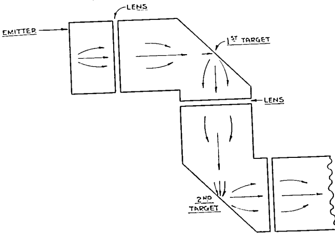
Fig. 14—L type multiplier.
