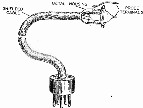
Fig. 13—A probe voltmeter using a miniature pentode.
