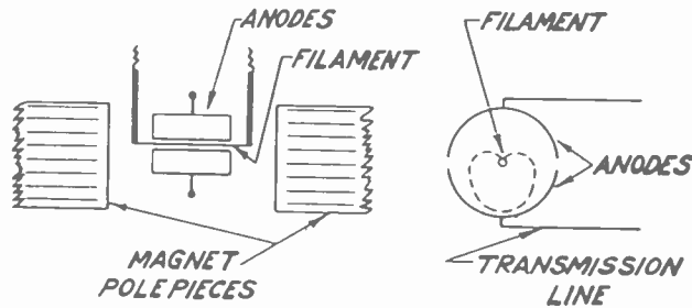
Fig. 2—Split-anode magnetron.
