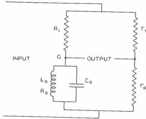
Fig. 1—Fundamental suppresser.
