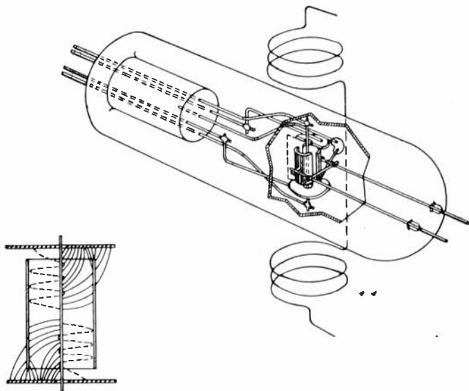
Fig. 3—End-plate magnetron.
