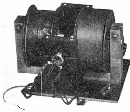
Fig. 12—Magnetron detector.
