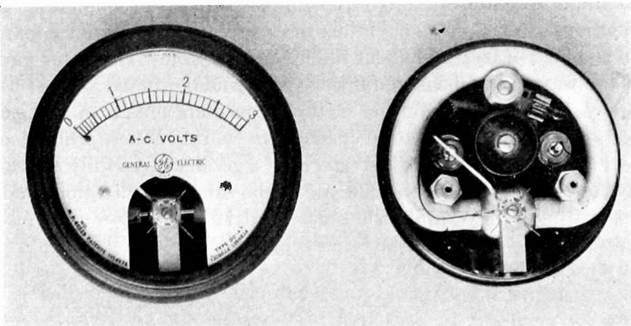
Fig. 15—Type DO-14x a-c miniature voltmeter.
