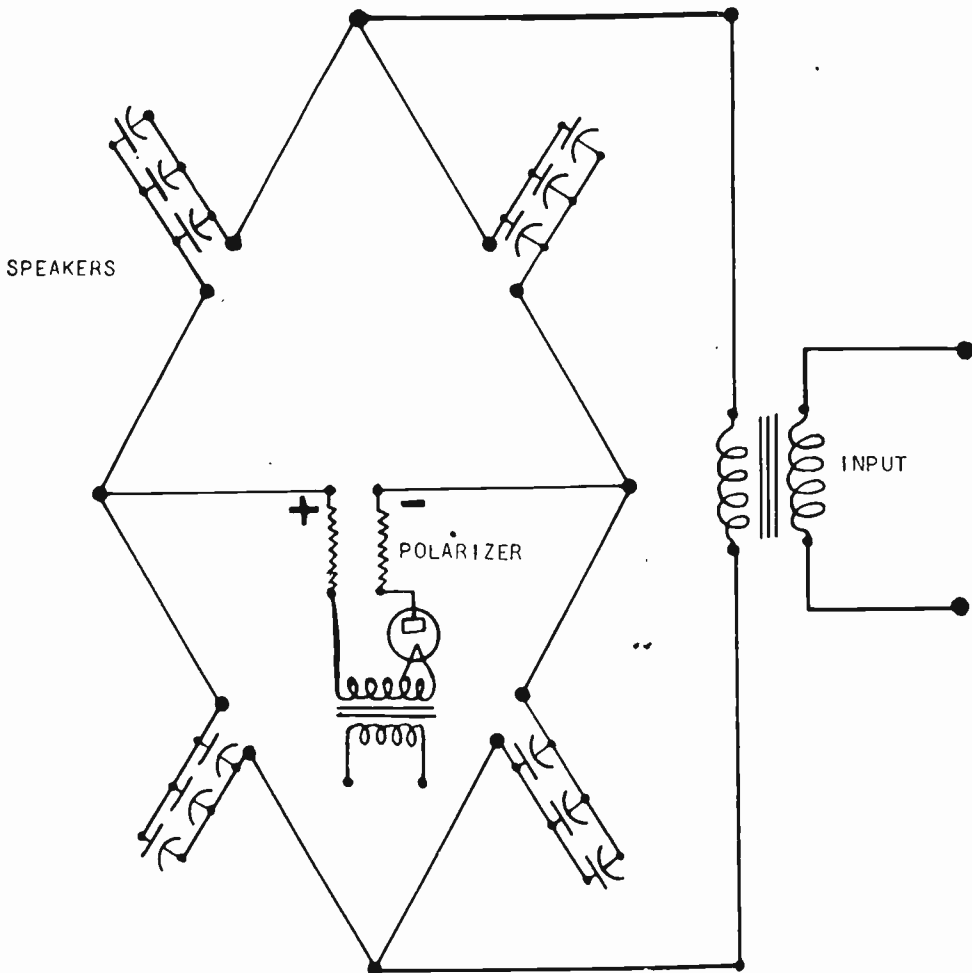
Fig. 6—Bridge circuit.
