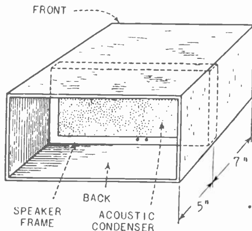
Fig. 4—Box baffle arrangement.
