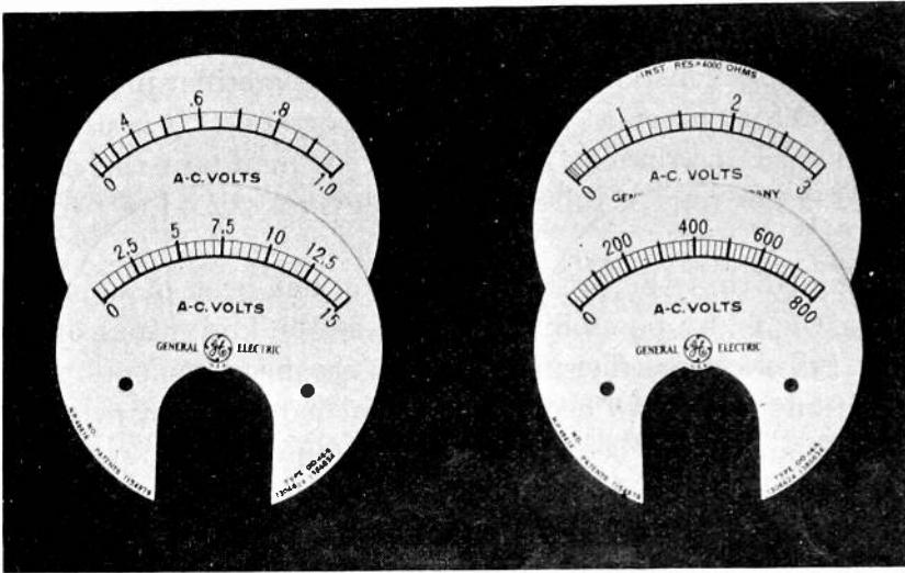
Fig. 14—Typical rectifier voltmeter scales.
