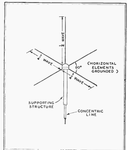
FIG. 3. THE GROUND-PLANE ANTENNA
