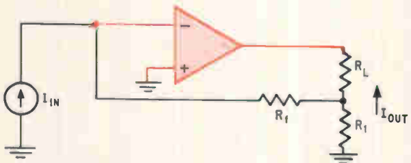
(d) CURRENT AMPLIFIER
