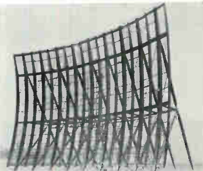
■ 25×16 meter scatter antenna
