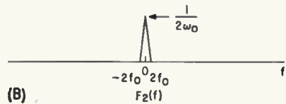
(B) F_2(f)
