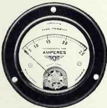
68 R. F. Ammeter
