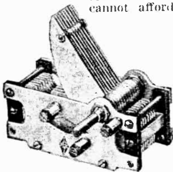
The New M. R. L. STRAIGHT LINE FREQUENCY C o n d e n s e r
