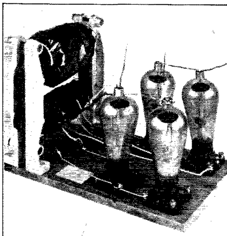
THE COMPLETE 3500-VOLT RECTIFIER
