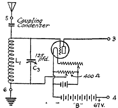
FIG. 2 THE R. F. AMPLIFIER
