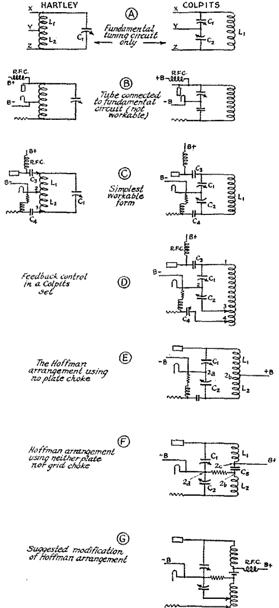
FIG. 10 COLPITTS CIRCUITS
