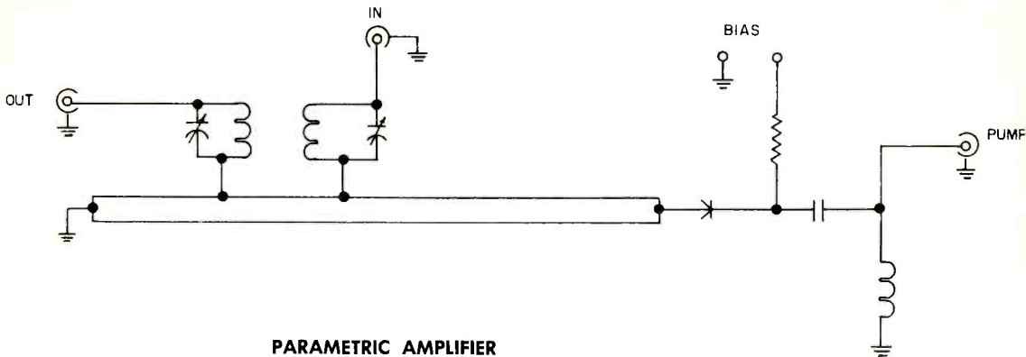
PARAMETRIC AMPLIFIER
