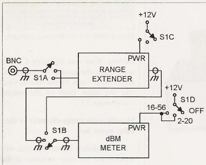
Fig. 8. Switch diagram.
