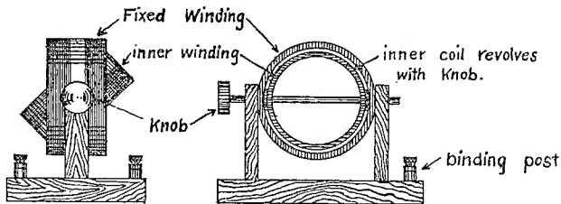
Fig. 85. Variometer.
