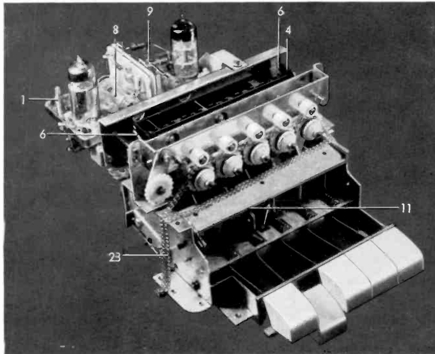
Bild 1 Gesamtansicht des GRUNDIG Stationstasten-Aggregats
