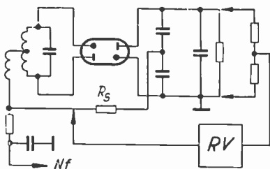
Ratio-detektor (unsymmetrischer Verhältnisleichtrichter)
