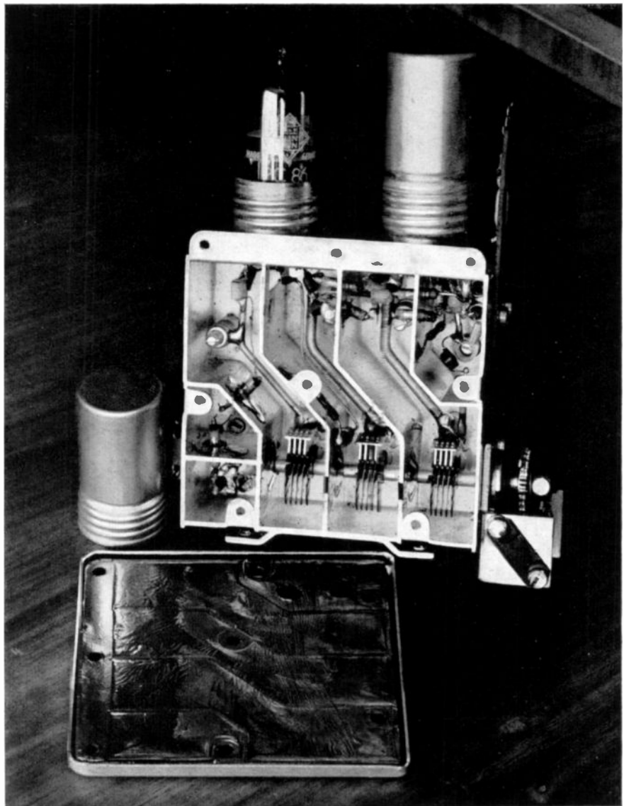
Bild 4 UHF-Teil geöffnet
