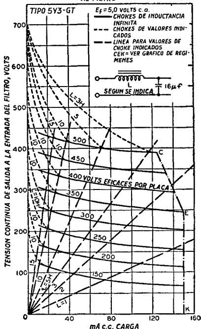
CARACTERISTICAS DE TRABAJO CIRCUITO DE ONDA COMPLETA CON CHOKE DE ENTRADA AL FILTRO
