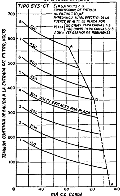
CARACTERISTICAS DE TRABAJO CIRCUITO DE ONDA COMPLETA CON CONDENSADOR DE ENTRADA AL FILTRO
