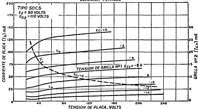
CARACTERÍSTICAS MEDIAS DE PLACA CONEXION PENTODO
