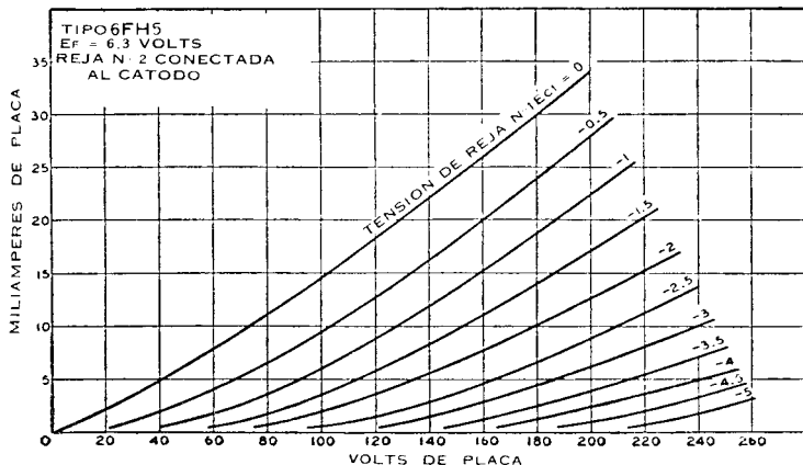
CARACTERISTICAS MEDIAS DE PLACA
