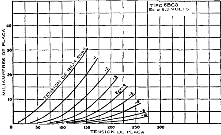
CARACTERÍSTICAS MEDIAS POR CADA UNIDAD
