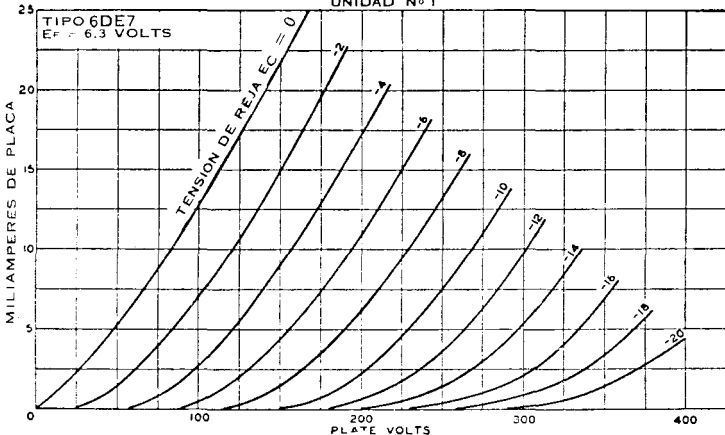
CARACTERISTICAS MEDIAS DE PLACA UNIDAD N° 1
