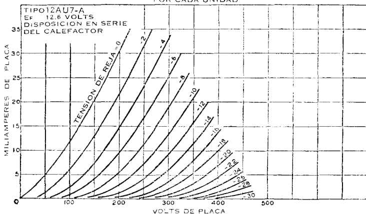
CARACTERISTICAS MEDIAS DE PLACA POR CADA UNIDAD
