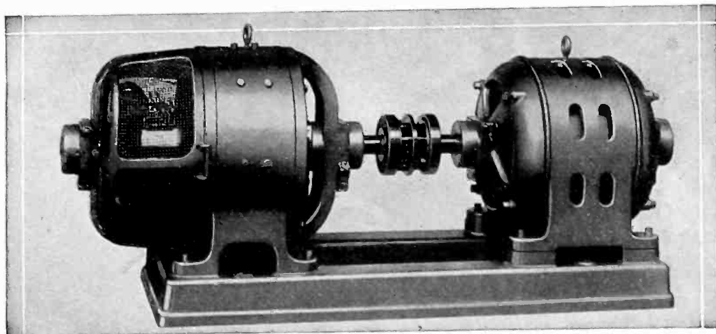
25 K. W. Motor Generator Set
