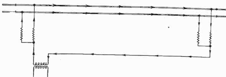
FIG. 3—LOOP CIRCUIT
