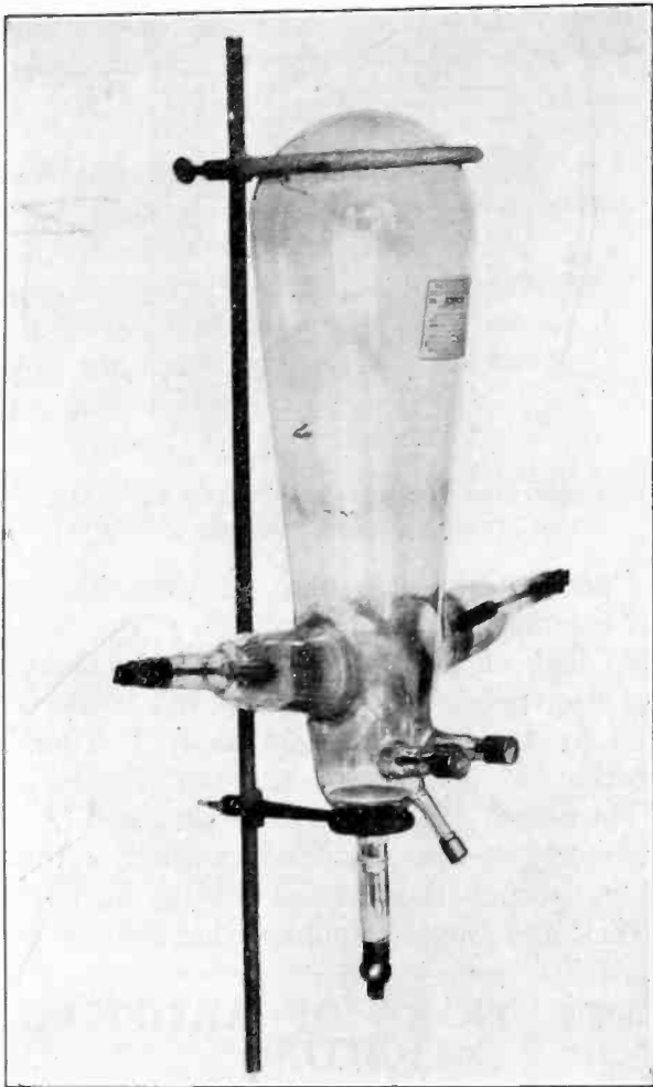
FIG. 15—150-VOLT MERCURY ARC RECTIFIER TUBE
